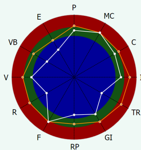
Круговые диаграммы
